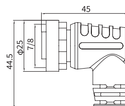
弯头插孔
