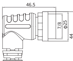
弯头插针
