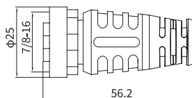
直头插孔
